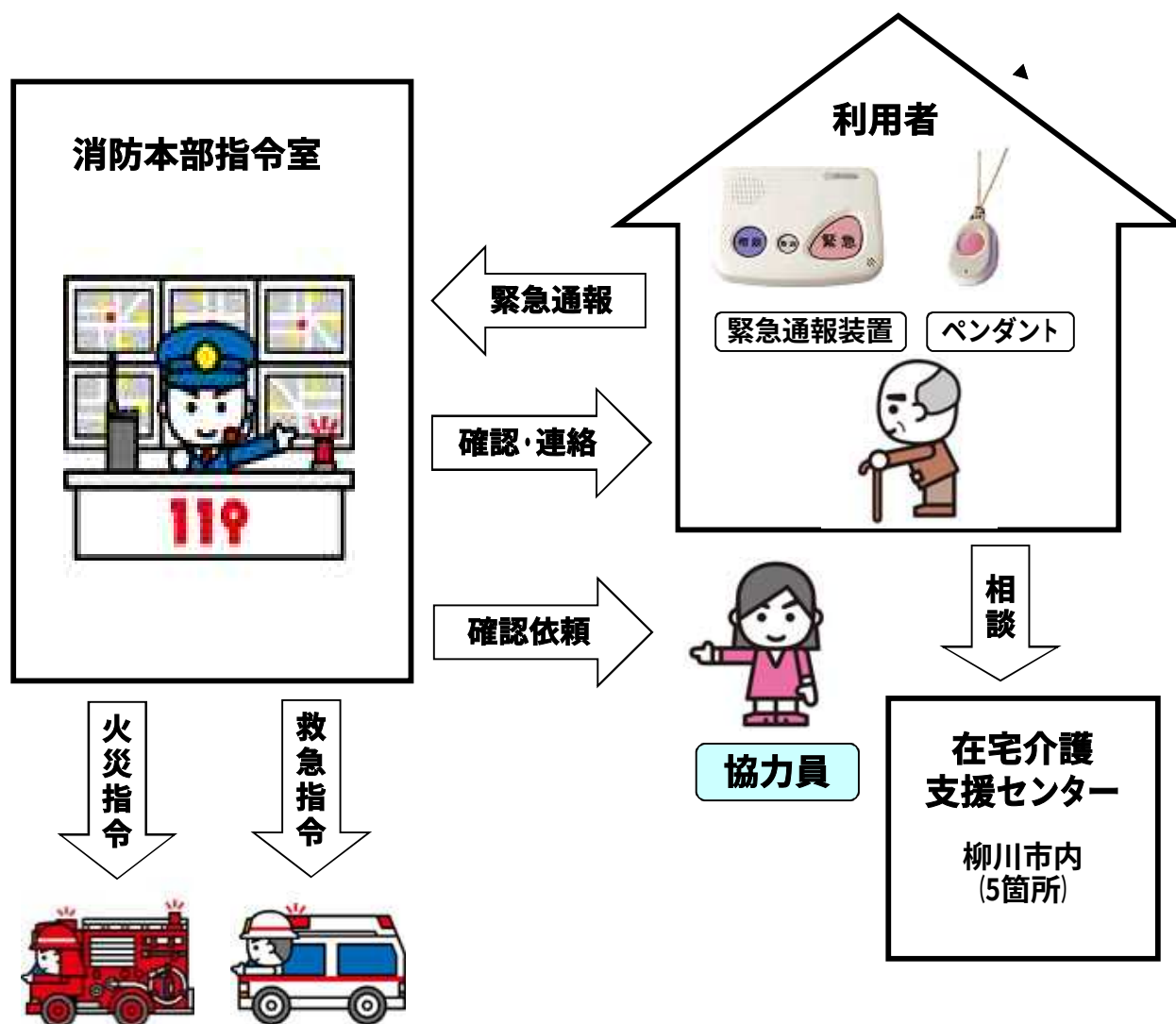
緊急通報装置の施設系統図
