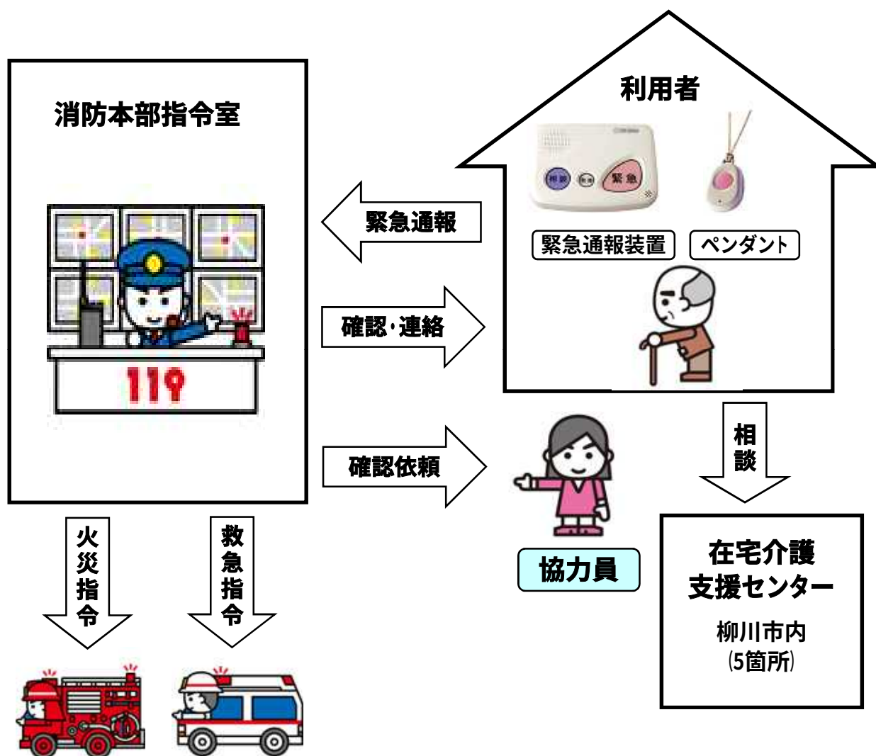
緊急通報装置の施設系統図
