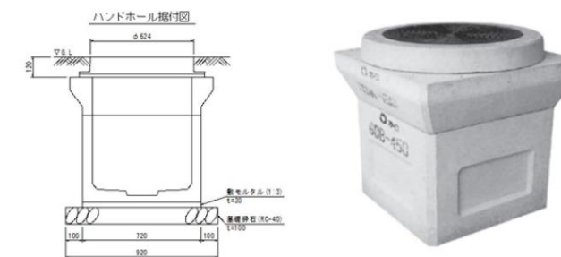
（ハンドホール参考図）
