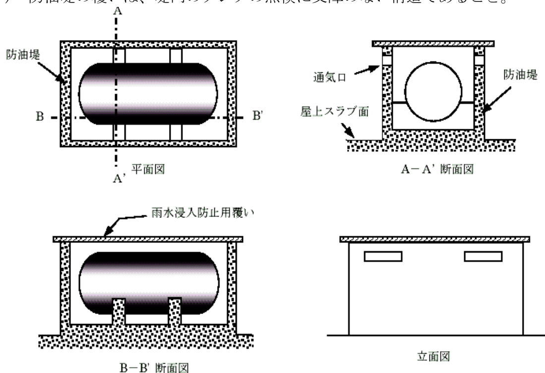
例図3 中継タンクの防油堤概略図
