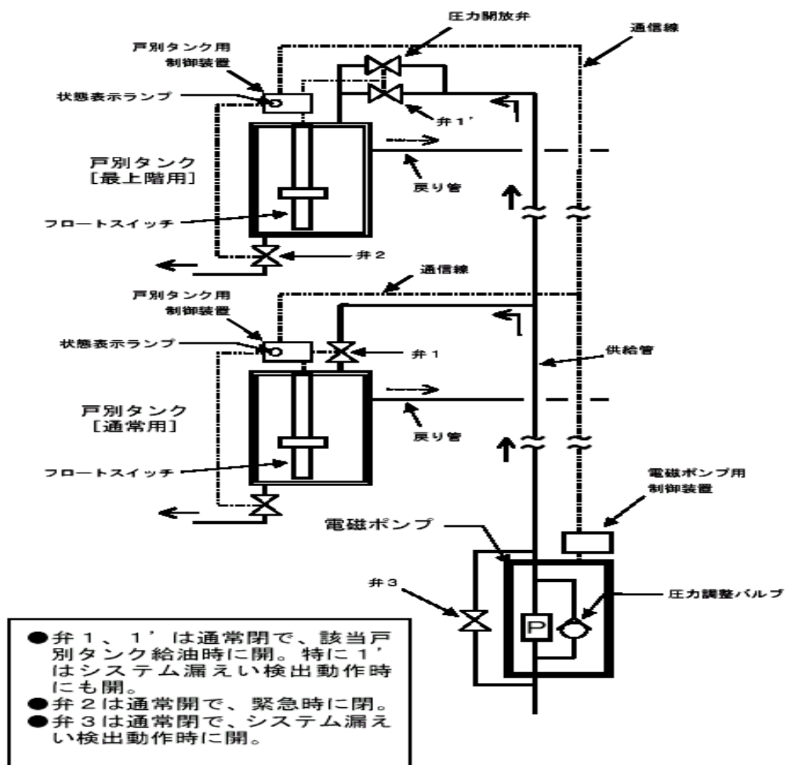
例図6－2 戸別タンクと電磁ポンプの詳細図（方式例2）
