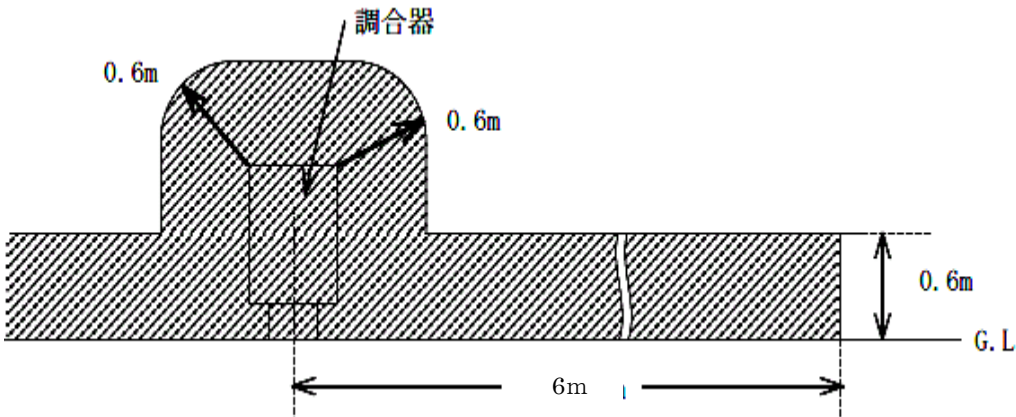
第18-6図 混合燃料調合器
