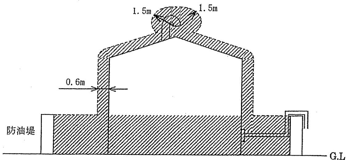
第18－3図 屋外タンク貯蔵所
