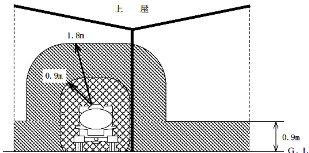
第18－2図 上屋を有するローリー積場
