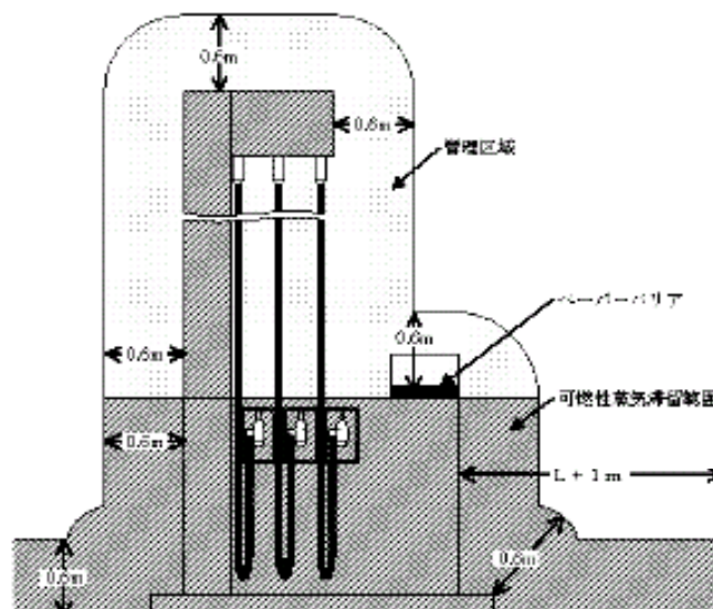
第18-4-4 図 地上式固定給油設備等 (可燃性蒸気流入防止構造)
