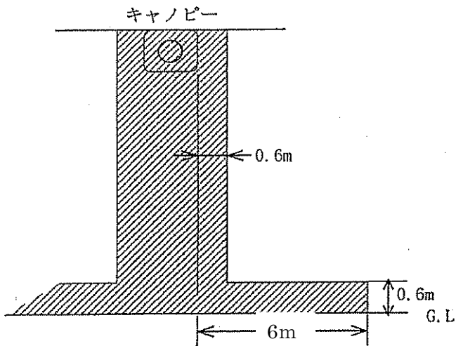
第18－5図 懸垂式固定給油設備（可燃性蒸気流入防止構造以外）
