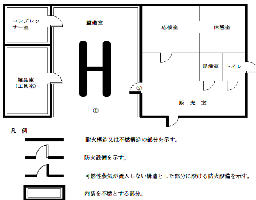
第12－17図 内部構造例
