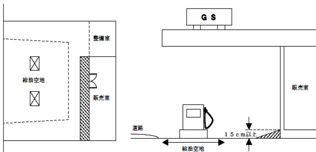
第12-18図 コンクリート製スロープ設置例
