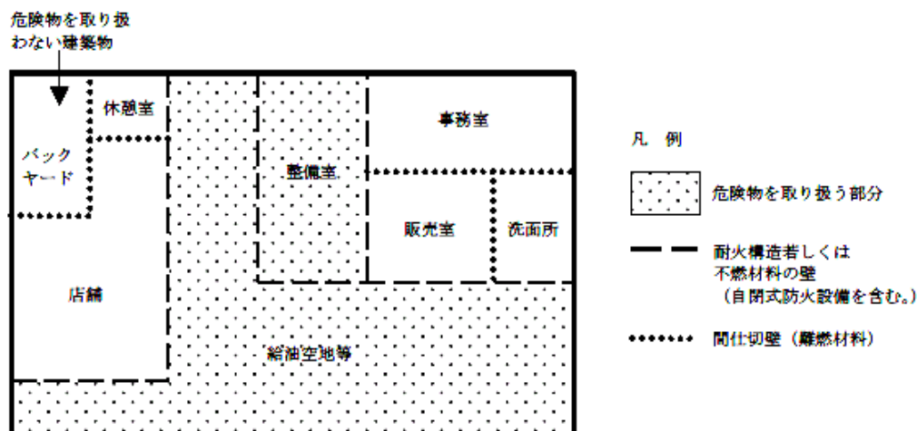
第12-15図 不燃材料以外の建築材料で造ることのできる間仕切壁の例
