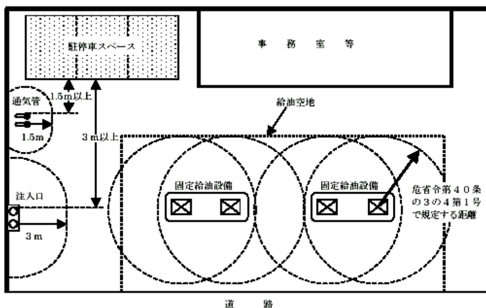
第12-31図 駐停車スペースの例
