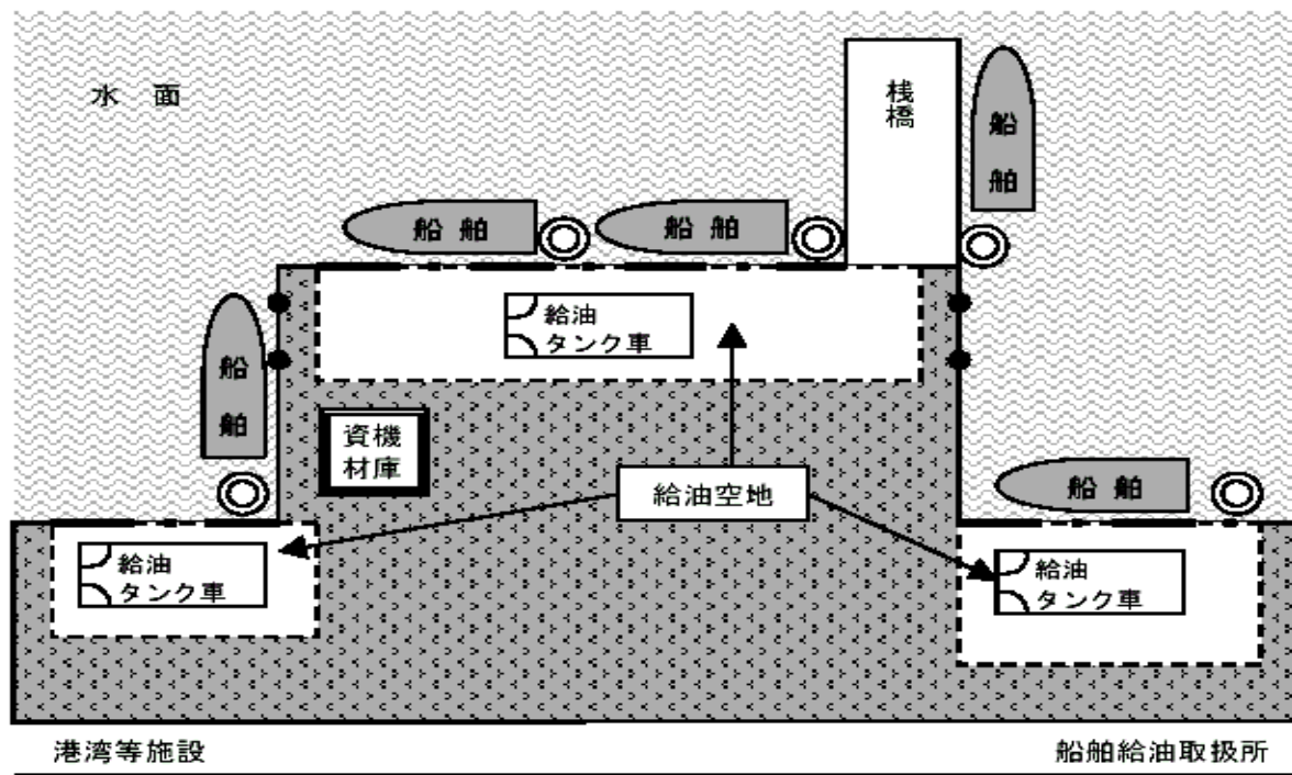
第12-45図 一の船舶給油取扱所に複数の給油空地を設ける場合の設置例
