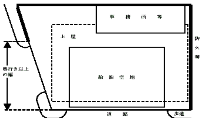
第12-34図 二方開放の例
