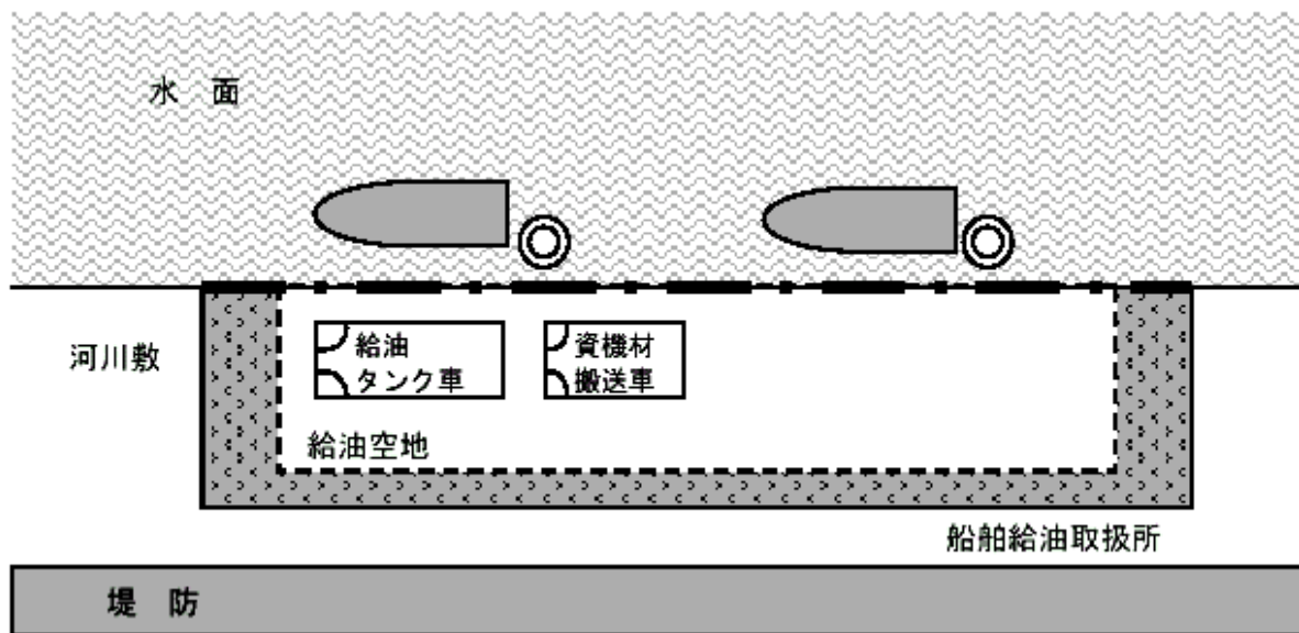
第12-46図 給油時に流出防止設備等の資機材を搬送する場合の設置例
