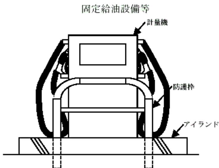
第12-37図 衝突防止措置の例
