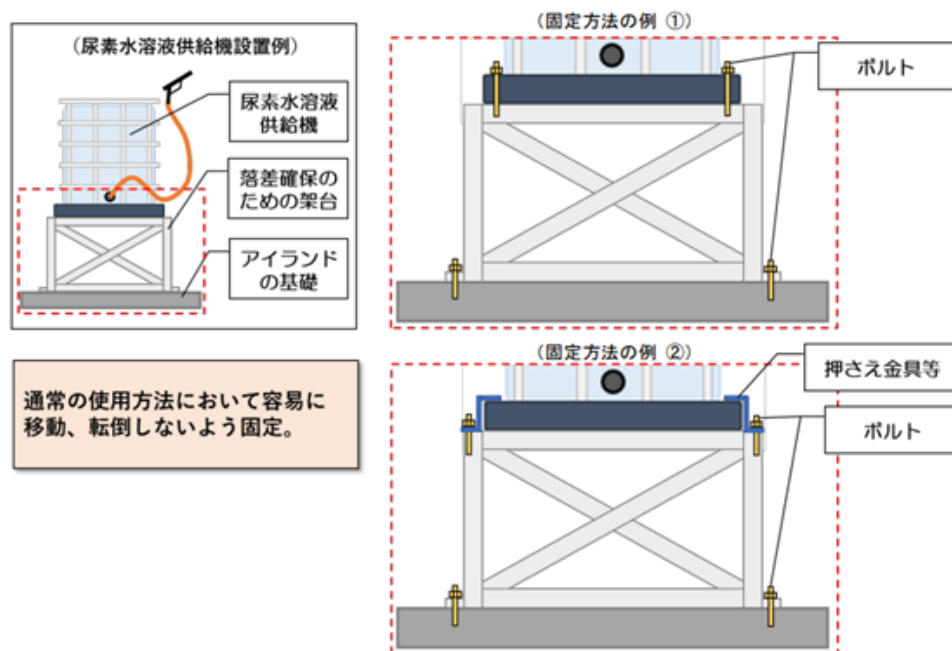
第12-28図 尿素水溶液供給機(重力により払い出すタイプ)
