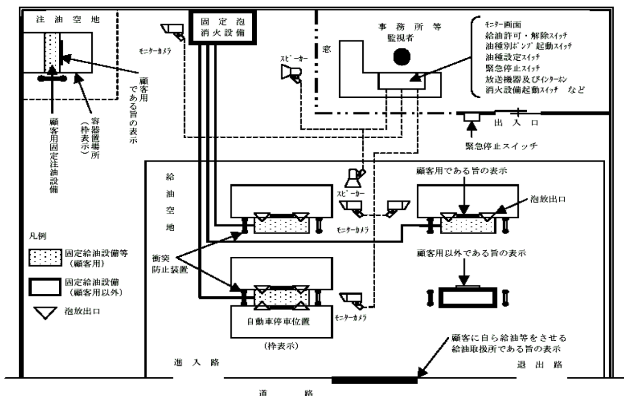
第12-54図 セルフ給油取扱所の設置例
