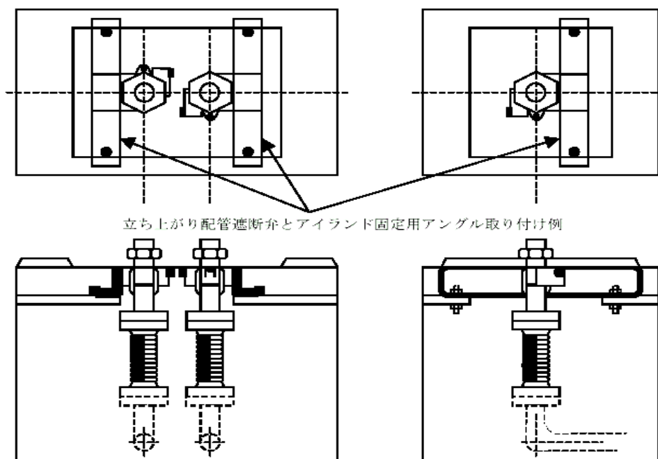
第12-52図 立がり配管遮断弁の取り付け例
