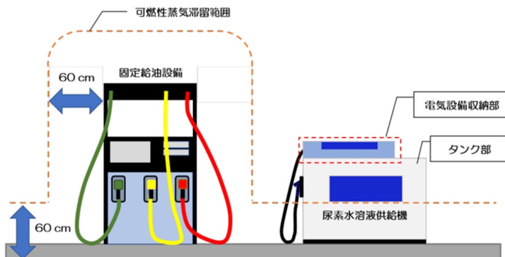
第12-27図 尿素水溶液供給機（電動ポンプにより払い出すタイプ）
