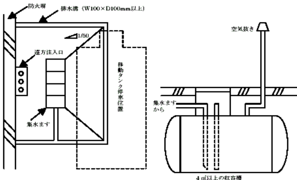
第12-42図 漏えい局限化措置の例
