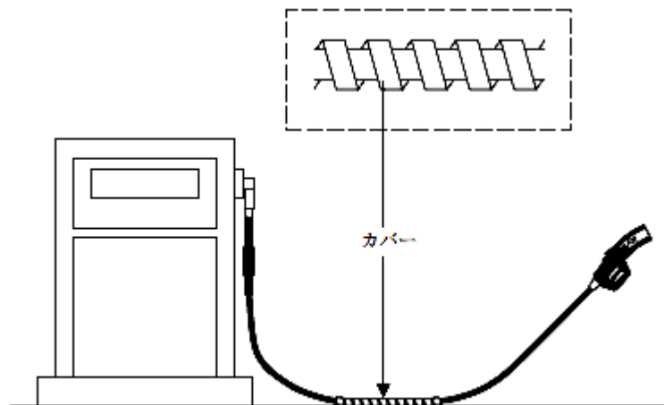
第12-23図 リング、カバーが取り付けられた給油ホース等
