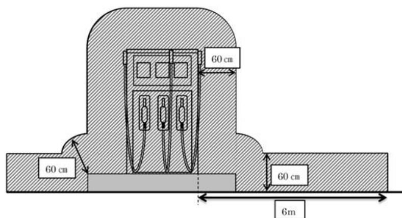
図 1 固定給油設備の周囲
