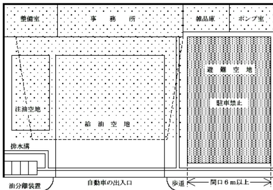
第12-35図 避難空地
