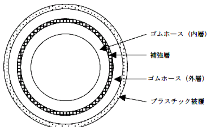
第12-24図 プラスチックで被覆された給油ホース等の構造（断面）
