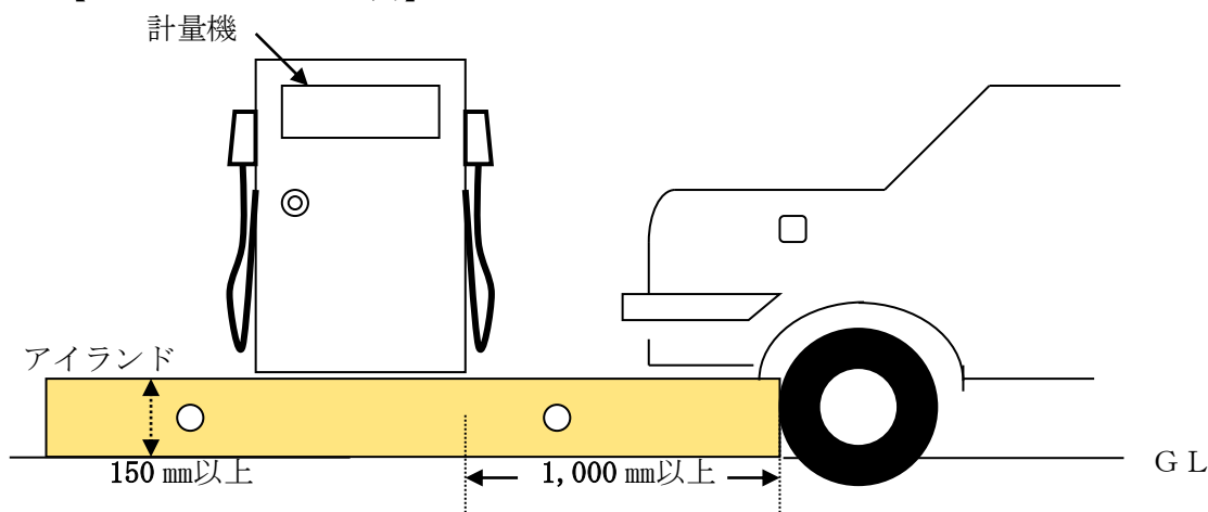
第12-50図 衝突防止措置の例
