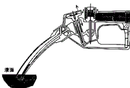
第12-49図 満量停止制御装置の構造例
