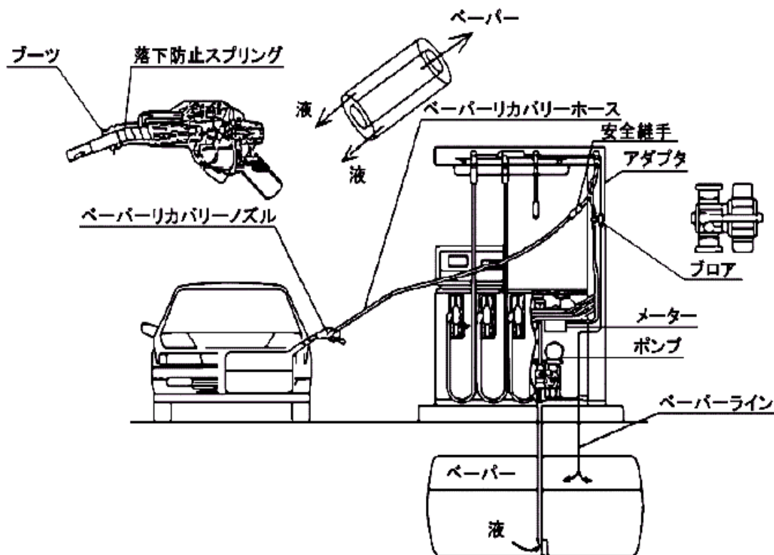
第12-48図 可燃性蒸気回収装置の構造例
