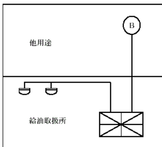
第12－40図 他用途に報知する設備の例
