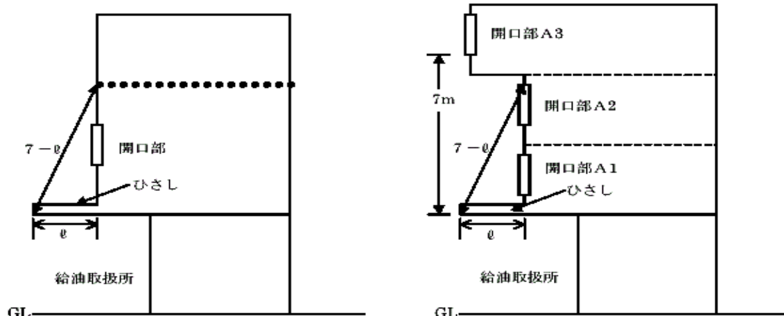
第12-43図 延焼防止上有効な屋根又はひさしの設置例
