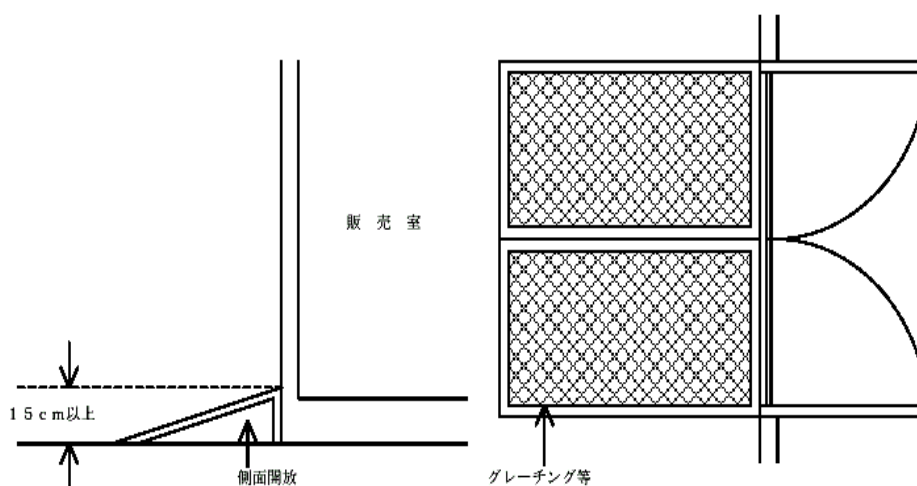
第12-19図 可燃性蒸気滞留防止構造例
