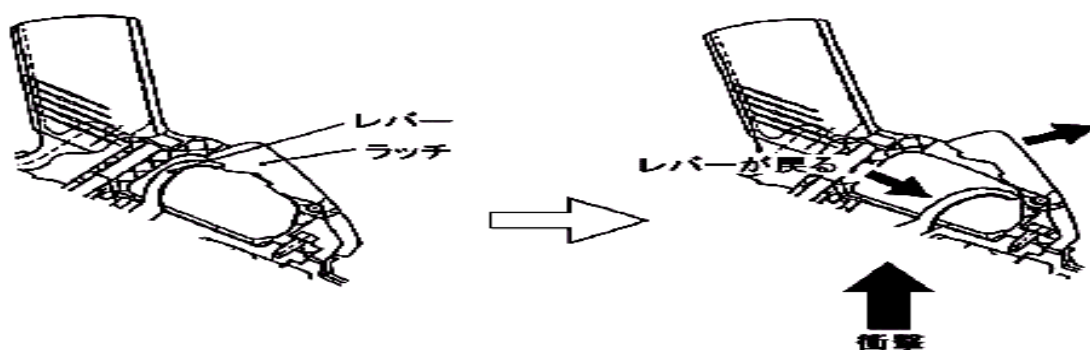
第12-47図 脱落時停止制御装置の構造例
